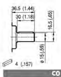
Coppia Max Max Torque 125 Nm
