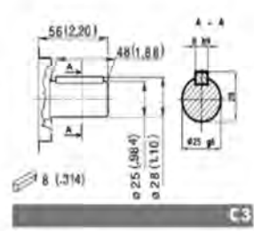
C3 Coppia Max Max Torque 380 Nm
