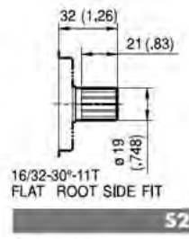
Coppia Max Max Torque 230 Nm
