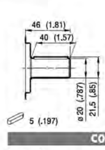
C0 Coppia Max Max Torque 265 Nm
