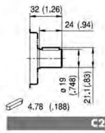
Coppia Max Max Torque 150 Nm
