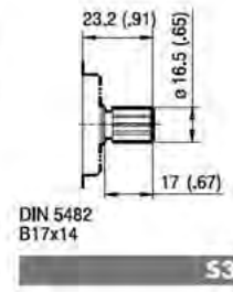
Coppia Max Max Torque 130 Nm
