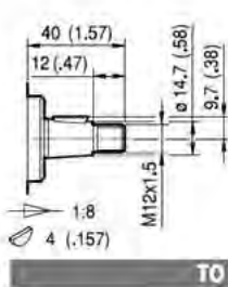
Coppia Max Max Torque 145 Nm
