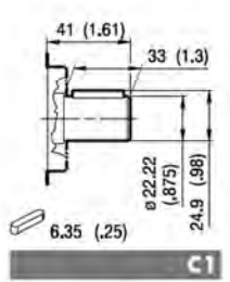
C1 Coppia Max Max Torque 295 Nm
